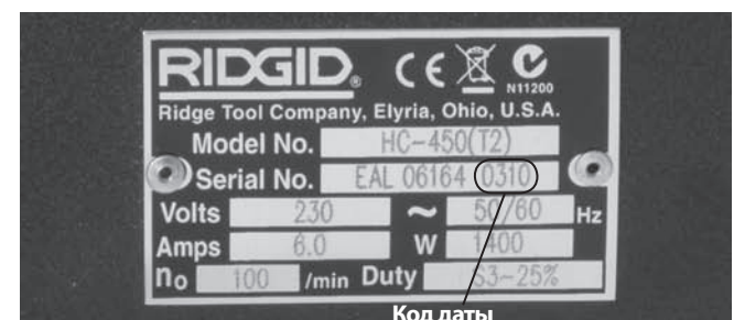
Рис. 3 – Серийный номер станка
