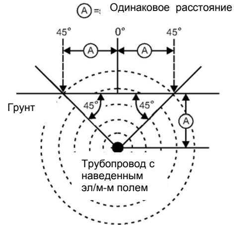
Рис. 8. Проверка искажения.
