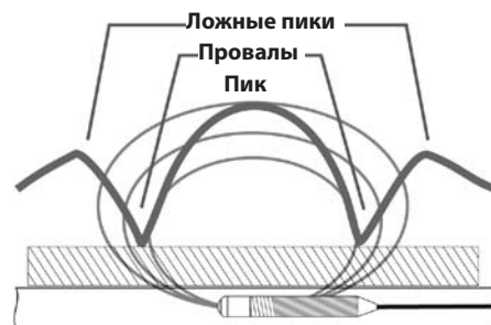
Рис. 35: Сигнал от зонда, который “видит” традиционный трассоискатель
