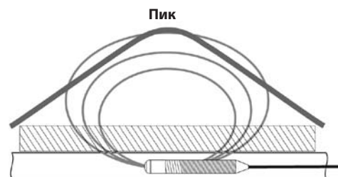
Рис. 36: Сигнал, который “видит” прибор NaviTrack® II
